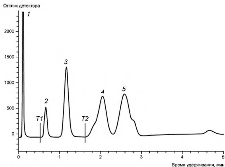
Детектор В (детектор по теплопроводности)
