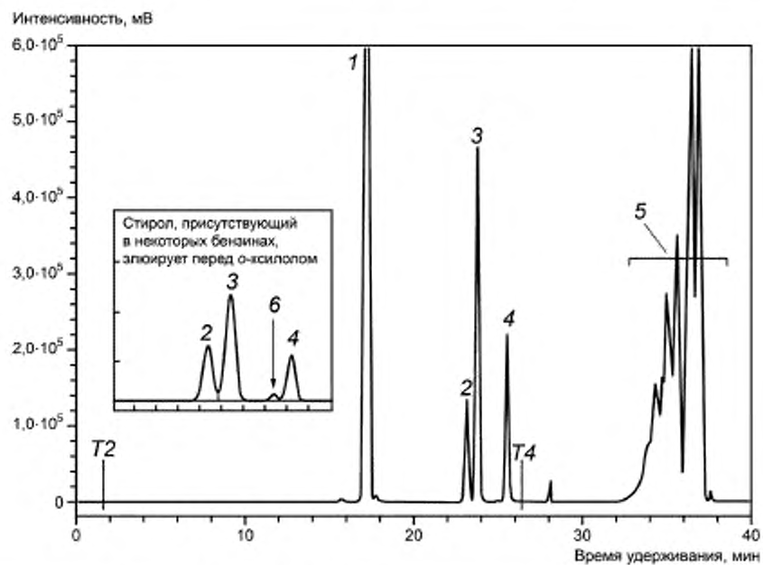
1 — 2-гексанон (внутренний стандарт); 2 — этилбензол; 3 — m/m -ксилол; 4 — o -ксилол; 5 — C_{9+} ароматические углеводороды; 6 — стирол
