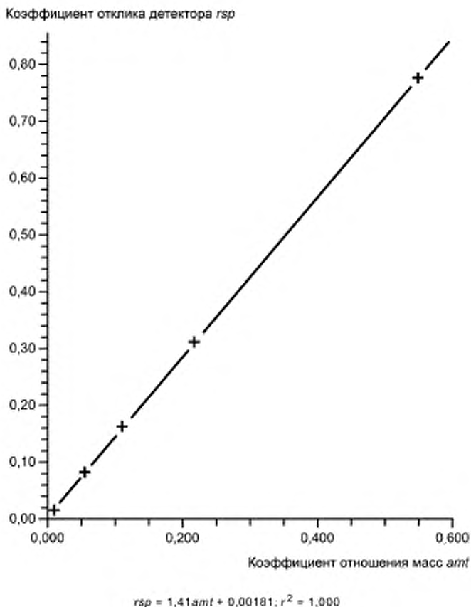
Рисунок 3 — Типовая калибровочная кривая для бензола
