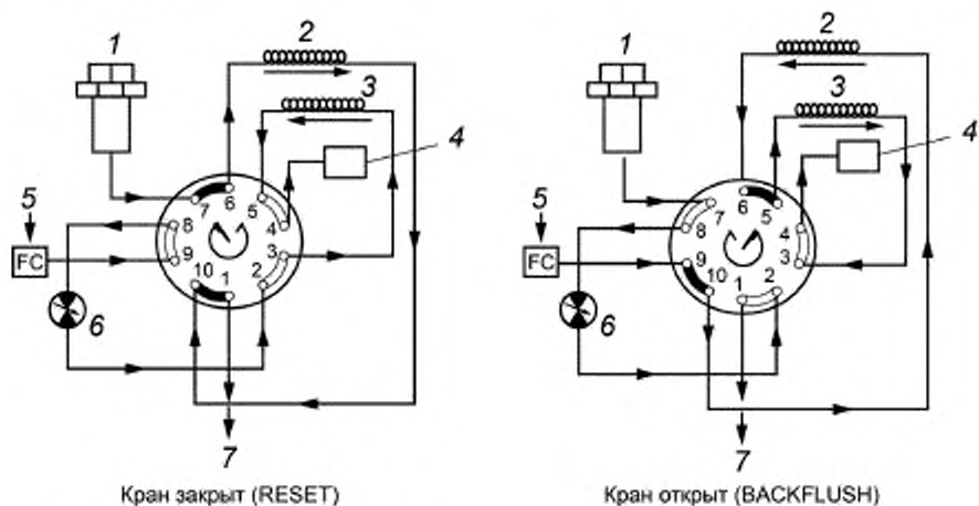
1 — инжектор; 2 — предколонка ТСЕР; 3 — капиллярная колонка; 4 — детектор А [пламенно-ионизационный детектор (FID)]; 5 — контроллер вторичного потока; 6 — регулируемый ограничитель; 7 — выпуск или детектор В [детектор по теплопроводности (TCD)]
