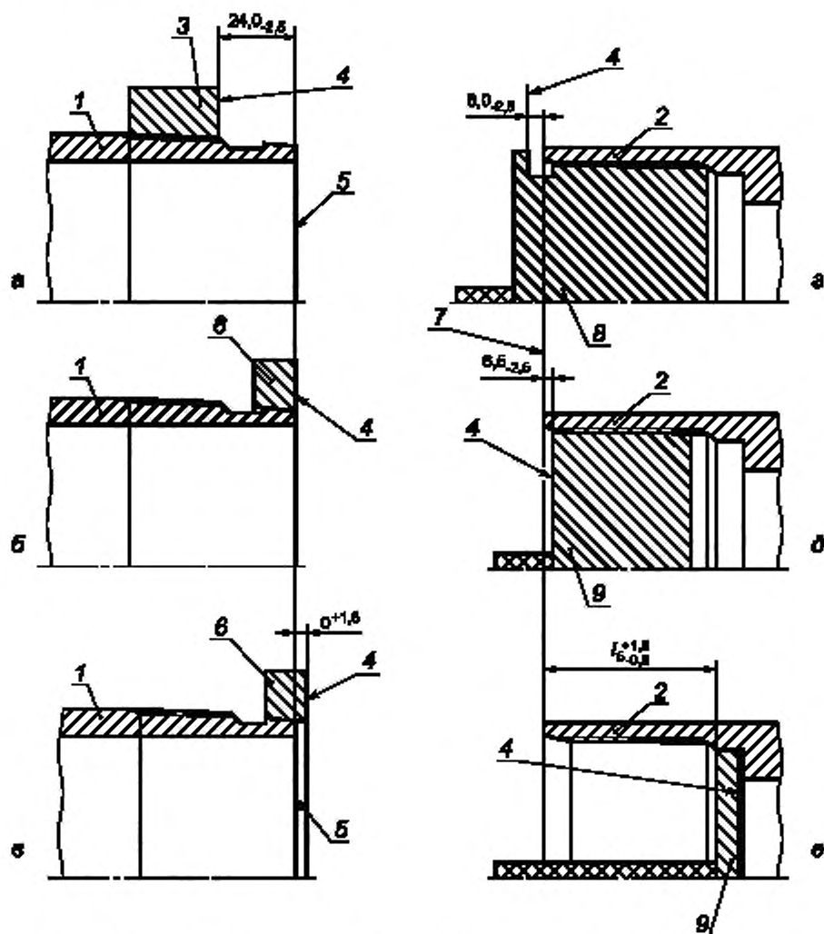
1 — труба; 2 — муфта; 3 — резьбовой и гладкий калибры-кольца; 4 — измерительная плоскость; 5 — плоскость торца трубы; 6 — гладкий калибр-кольцо; 7 — плоскость торца муфты; 8 — резьбовой калибр-пробка; 9 — гладкий калибр-пробка; l_5 — расстояние от торца муфты до конца сбега резьбы
