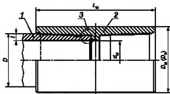
1 — труба; 2 — муфта; 3 — узел уплотнения металл-металл; D — наружный диаметр трубы, D_M — наружный диаметр обычной муфты; D_с — наружный диаметр специальной муфты; d_в — внутренний диаметр муфты. L_M — длина муфты. t — толщина стенки трубы
