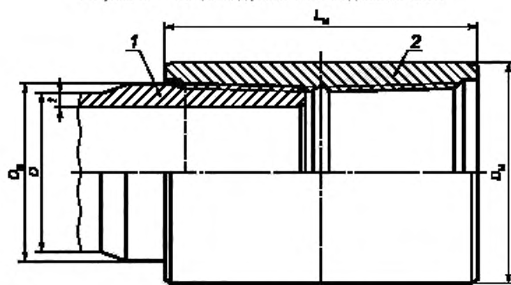
1 — труба; 2 — муфта; D — наружный диаметр трубы; D_n — наружный диаметр высаженного конца трубы; D_M — наружный диаметр муфты; L_M — длина муфты; t — толщина стенки трубы
