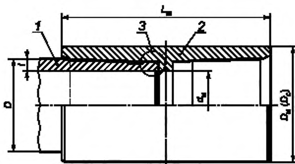
1 — труба; 2 — муфта; 3 — узел уплотнения металл-металл; D — наружный диаметр трубы.
