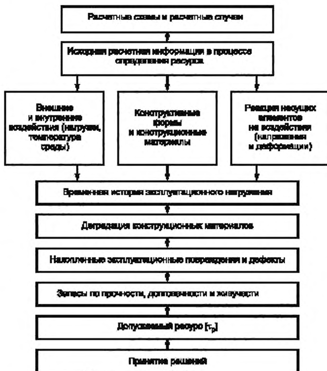
Рисунок 2 — Блок-схема определения ресурса
