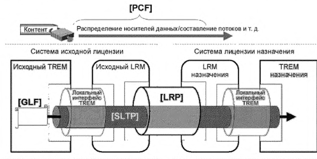
Рисунок 5 — Основная модель взаимодействия при защите контента
