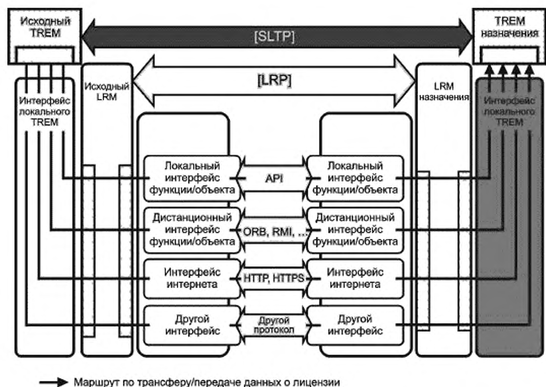
Рисунок 6 — Модель реализации взаимодействия
