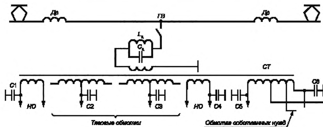
Рисунок 7.2 — Схема подавления помех для ЭПС переменного тока
