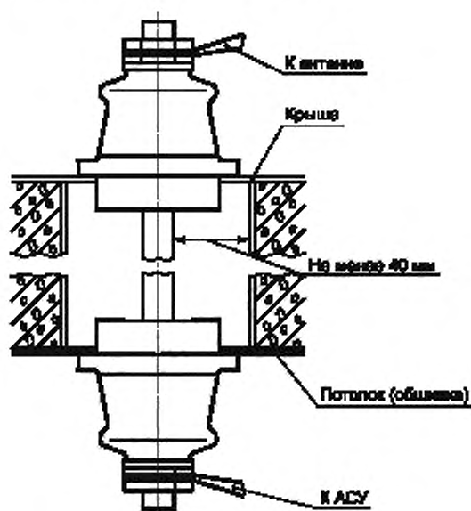
Рисунок 5.2 — Антенные вводы, собранные из двух проходных изоляторов
