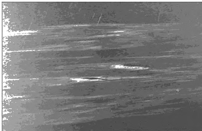
Рисунок А.40 — Включения в лаковом (эмалевом) покрытии
