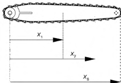
Рисунок 2 — Положения стопорного механизма пильной цепи
