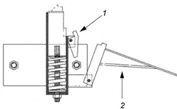
Рисунок А.2 — Стопорное устройство пильной цепи в разблокированном положении
