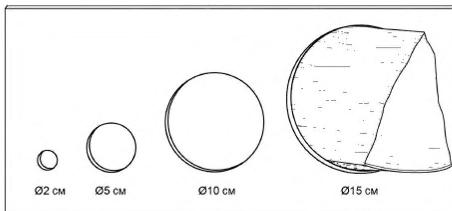
Рисунок В.2 — Измерение диаметра дров 2)
