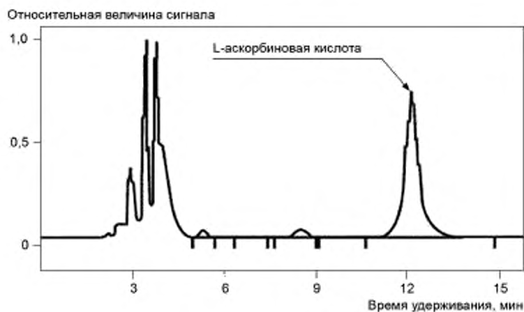
Рисунок А.1 — Пример хроматограммы при определении аскорбиновой кислоты в апельсиновом соке с помощью ВЭЖХ (время удерживания: t_{\text{рет}} = 11,953 мин)
