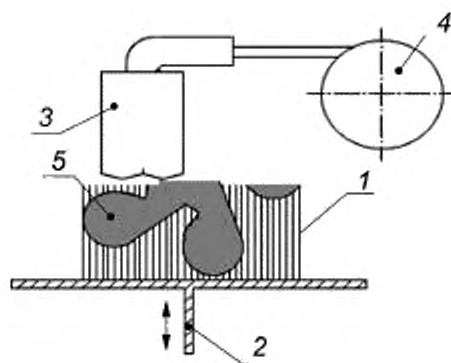
Рисунок 4 — Схема двух типов процесса синтеза на подложке
