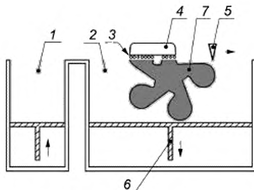
1 — система подачи порошка; 2 — порошкообразный материал, распределенный в ванне; 3 — жидкая связующая составляющая; 4 — дозирующее устройство, включая подключение к системе подачи связующего составляющего; 5 — устройство распространения порошка; 6 — строительная платформа и подъемник; 7 — получаемый продукт
