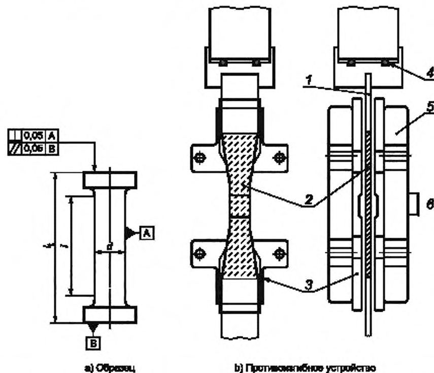
1 — нагрузочный стержень; 2 — образец; 3 — неподвижные боковые направляющие; 4 — уплотнительное кольцо; 5 — рама; 6 — свободная длина l — длина узкой параллельной части; l_1 — общая длина
