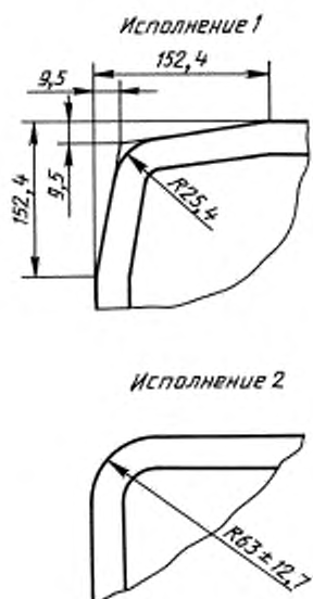
Рисунок 5 — Размеры основания (вид сверху)
