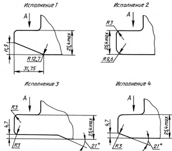
Рисунок 4 — Размеры основания (вид сбоку)
