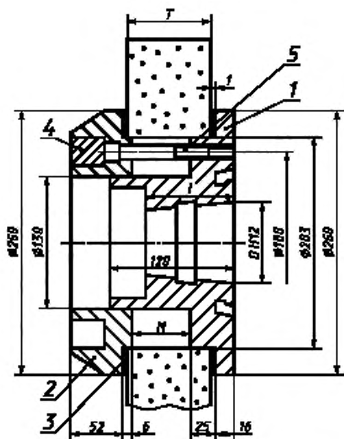
1 — неподвижный фланец; 2 — подвижный фланец; 3 — прокладка; 4 — сегмент; 5 — винт M16-6g × 56.029 по ГОСТ 11738
