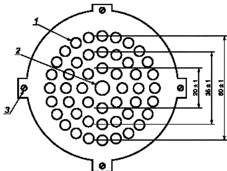
Рисунок 5 — Перфорированная пластина зонда зажигания
