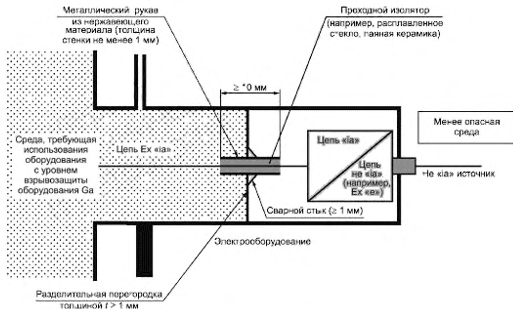
Рисунок 1 — Пример газонепроницаемой разделительной перегородки с проходным изолятором
