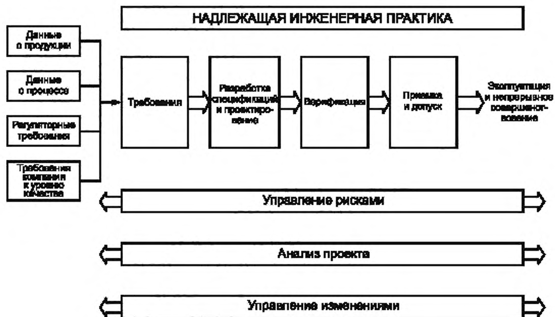
Рисунок 1 — Процесс разработки спецификаций, проектирования и верификации
