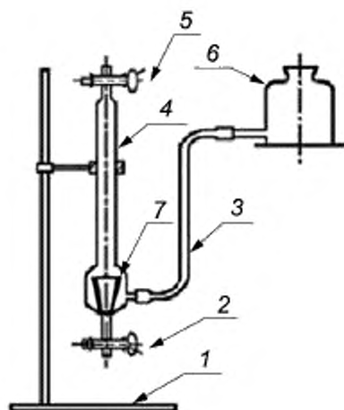
1 — штатив; 2 — кран В; 3 — шланг; 4 — градуированная трубка; 5 — кран А, 6 — резервуар с кислотой; 7 — контейнер
