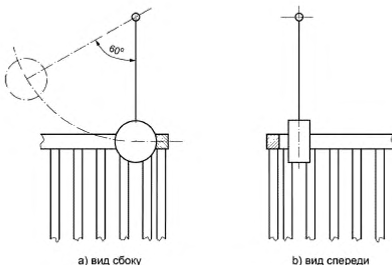
Рисунок 11 — Схема испытания на удар угла кровати
