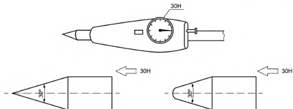
Рисунок 1 — Примеры измерительных конусов
