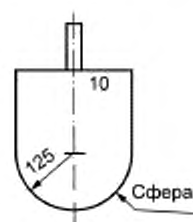
Рисунок 2 — Сбрасываемый ударник
