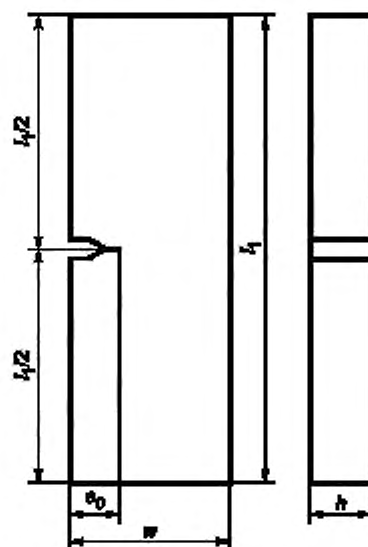
w — ширина; l_1 — длина; h — толщина; a_0 — начальная длина трещины
