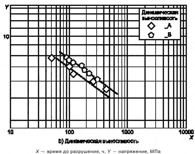
Рисунок А.2 — Пример динамической и статической усталостной выносливости двух материалов, проявляющих противоположное поведение
