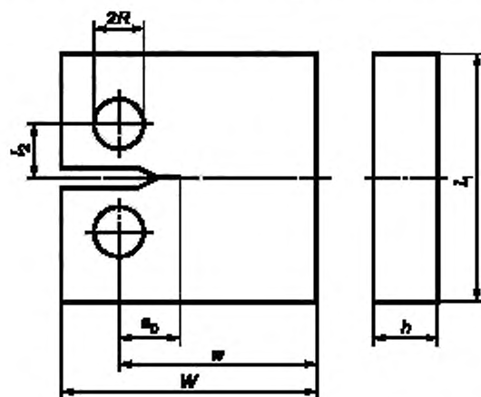
w — эффективная ширина; W — общая ширина; l_1 — длина; l_2 — расстояние между центрами отверстий для шпилек, расположенных симметрично к плоскости трещины в пределах \pm 0,005 w ; R — радиус отверстия под шпильку; h — толщина; a_0 — начальная длина трещины
