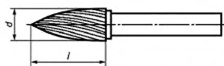
Рисунок 6 — Борфреза типа G
