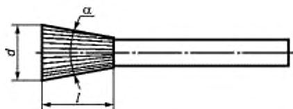
Рисунок 11 — Борфреза типа N
