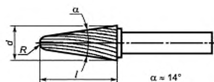
Рисунок 9 — Борфреза типа L
