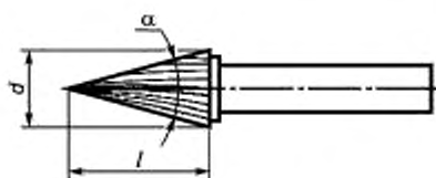
Рисунок 10 — Борфреза типа M
