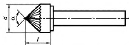
Рисунок 8 — Борфреза типов J и K
