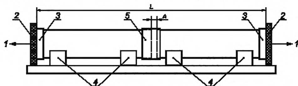
1 — осевое давление, воздействующее на образец для испытаний; 2 — оснастка испытательного стенда; 3 — торцевая заглушка; 4 — опоры; 5 — испытываемое соединение; А — общий вырыв; L — общая эффективная длина
