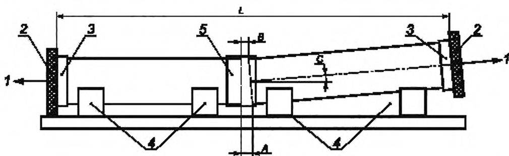
1 — осевое давление, воздействующее на образец для испытаний; 2 — оснастка испытательного стенда; 3 — торцевая заглушка; 4 — опоры; 5 — испытываемое соединение; А — общий вырыв; В — вырыв; С — угловое смещение; L — общая эффективная длина
