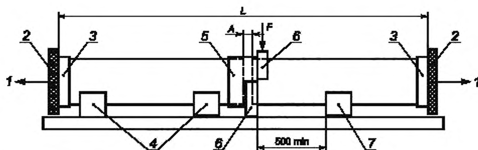
1 — осевое давление, воздействующее на образец для испытаний; 2 — оснастка испытательного стенда; 3 — торцевая заглушка; 4 — опоры; 5 — испытуемое соединение; 6 — хомут; 7 — опора «R»; A — общий вырыв, L — общая эффективная длина; F — сила смещения
