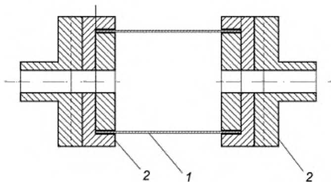
1 — образец; 2 — приспособление
