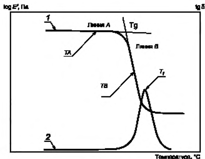
1 — график логарифма динамического модуля упругости E' ; 2 — график тангенса угла механических потерь \tan \delta ; T_i — температура пика тангенса угла механических потерь
