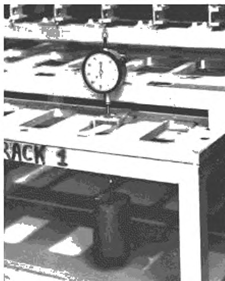
Рисунок 2 — Устройство для испытания на ползучесть при изгибе
