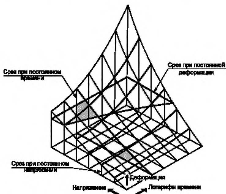
Рисунок Х4.1 — Постоянные координаты «напряжения—деформации—времени»
