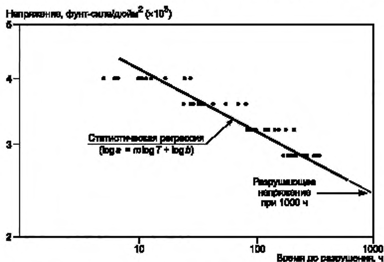
Рисунок 5 — Кривая логарифмической зависимости времени разрушения (механического разрушения)
