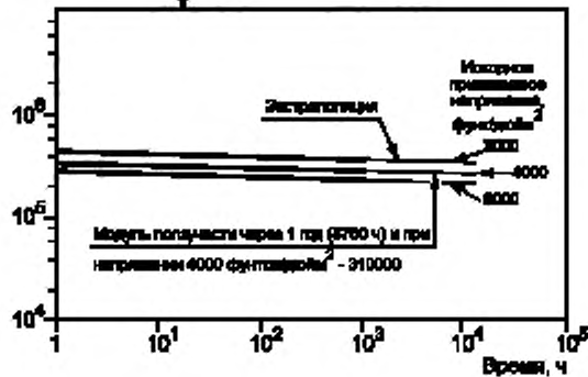
Рисунок 3 — Модуль ползучести 30% полибутилентерафтала, армированного стекловолокном, при 212° F, экстраполированный для получения расчетного модуля для точки 1 год
