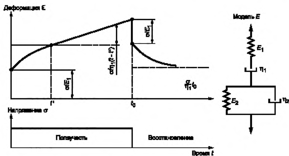
Рисунок Х6.3 — Четырехэлементная модель
