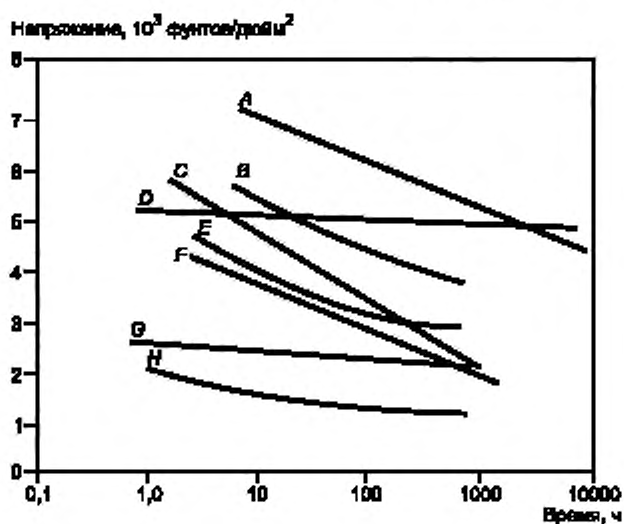
A — стиролакрилонитрил при 23 °С; B — эпоксидный КМ при 120 °С; C — 30 %-ный нейлон, армированный стекловолокном (сухой) при 120 °С; D — 30 %-ный полибутилентерефталат, армированный стекловолокном, при 150 °С; E — фенольный КМ с минимальным наполнителем при 120 °С; F — ацеталь при 80 °С; G — ударпрочный полистирол при 23 °С; H — алидный КМ при 120 °С
