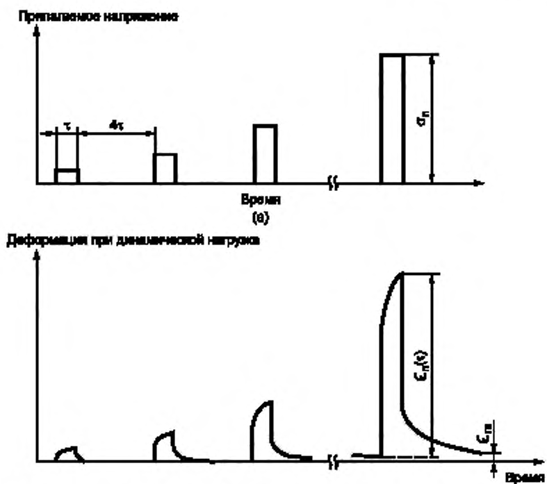
Деформация при растяжении
