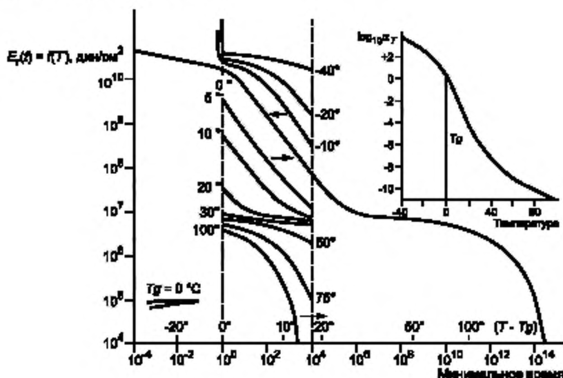
Рисунок X5.2 — Обобщающая кривая снятия напряжения
