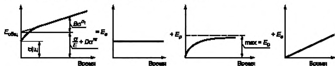
Рисунок Х6.2 — Кривая ползучести (три части)
