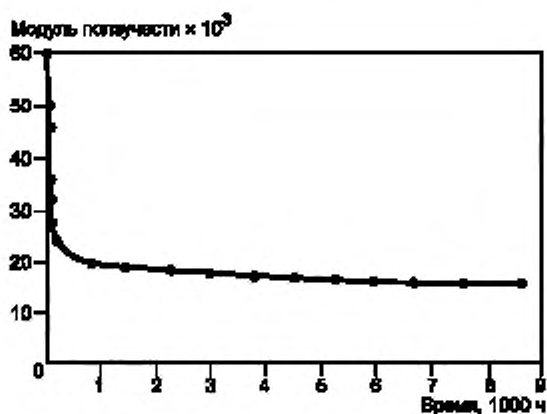
Рисунок X2.3 — Зависимость модуля ползучести от времени
