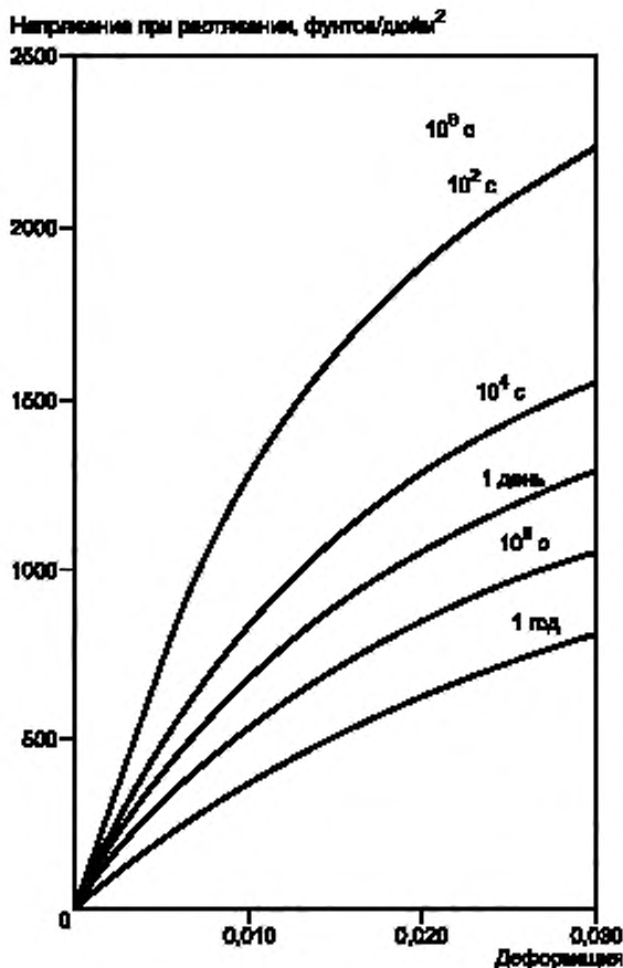
Рисунок X4.4 — Постоянные временные вертикальные разрезы для рисунка X4.3 (изохронные разрезы)
