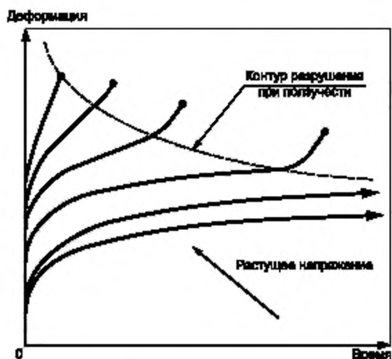
Рисунок X3.4 — Контур разрушения при ползучести
