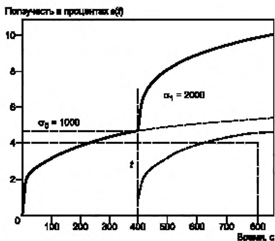
Рисунок X5.1 — Принцип Больцмана
