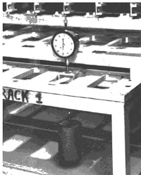
Рисунок А.1 — Испытательный стенд
