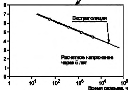
Рисунок 1 – Разрушение стиралакрило- нитрила при ползучести при 73 °F, экстра- полированное для получения расчетного напряжения для точки 5 лет
