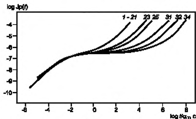
Рисунок X5.3 — Кривая податливости
