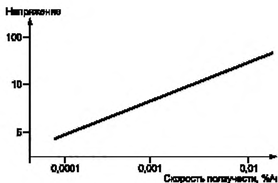
Рисунок Х3.2 — Прочность при ползучести
