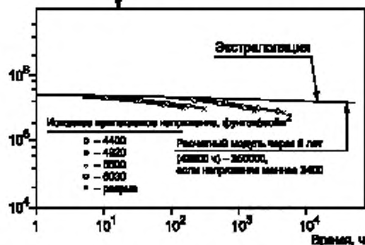
Рисунок 2 – Модуль ползучести стиралакрило- нитрила при ползучести при 73 °F, экстраполированное для точки получения расчетного модуля для точки 5 лет
