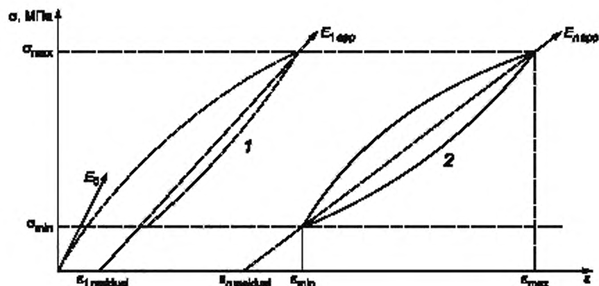
Рисунок 4 — Знакопостоянный цикл нагружения
