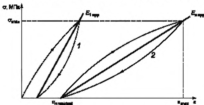
1 — первый цикл нагружения; 2 — n -й цикл нагружения
