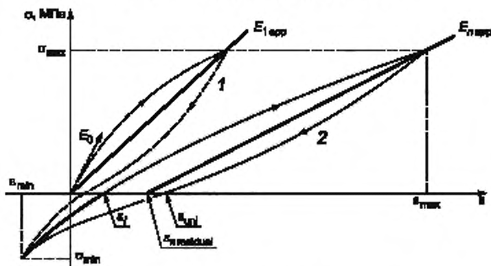
1 — первый цикл нагружения; 2 — n -й цикл нагружения
