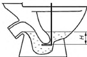
H — высота водяного затвора
