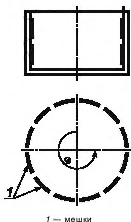
Рисунок 1 — Расположение мешков в барабане центрифуги
