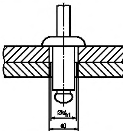
a) Увеличенное отверстие с зазором.
