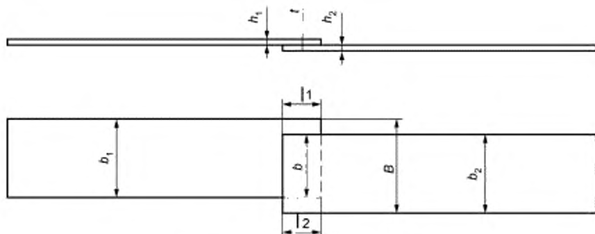
Рисунок 4 — Схема замера образца
