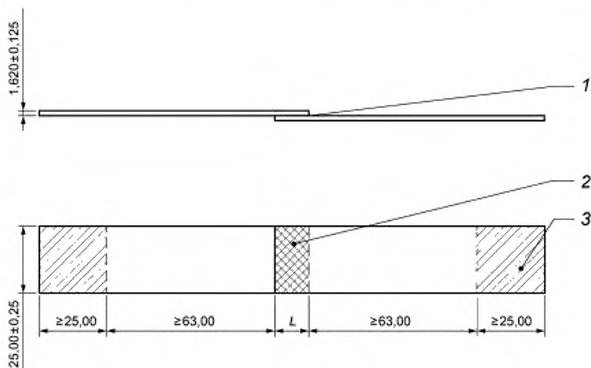
Рисунок 1 — Форма и размеры образца
