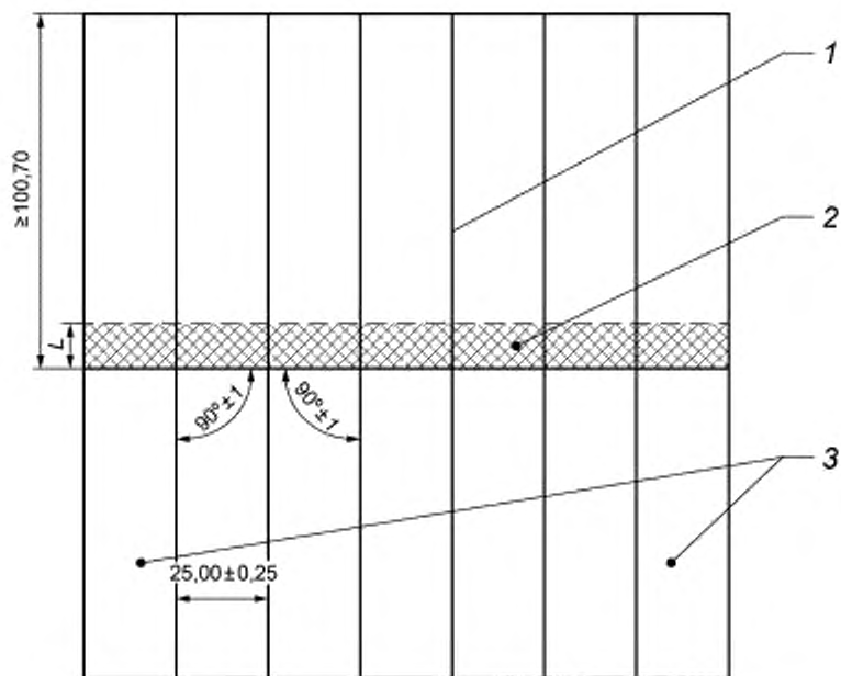
1 — линии разреза; 2 — зона нахлестки; 3 — края панелей
