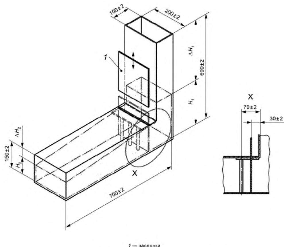
Рисунок 1 — Типовая конструкция L-образного короба с предусмотренными размерами
