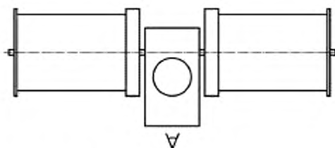
д) лебедка двухбарабанная симметричная
