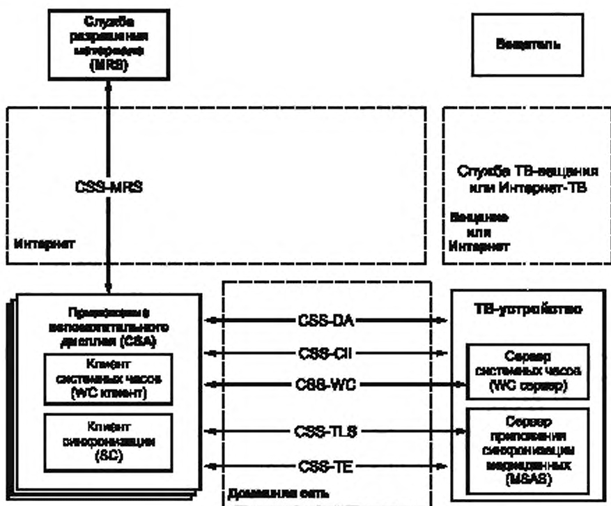
Рисунок 3 — Интерфейсы внутри составной поставляемой услуги
