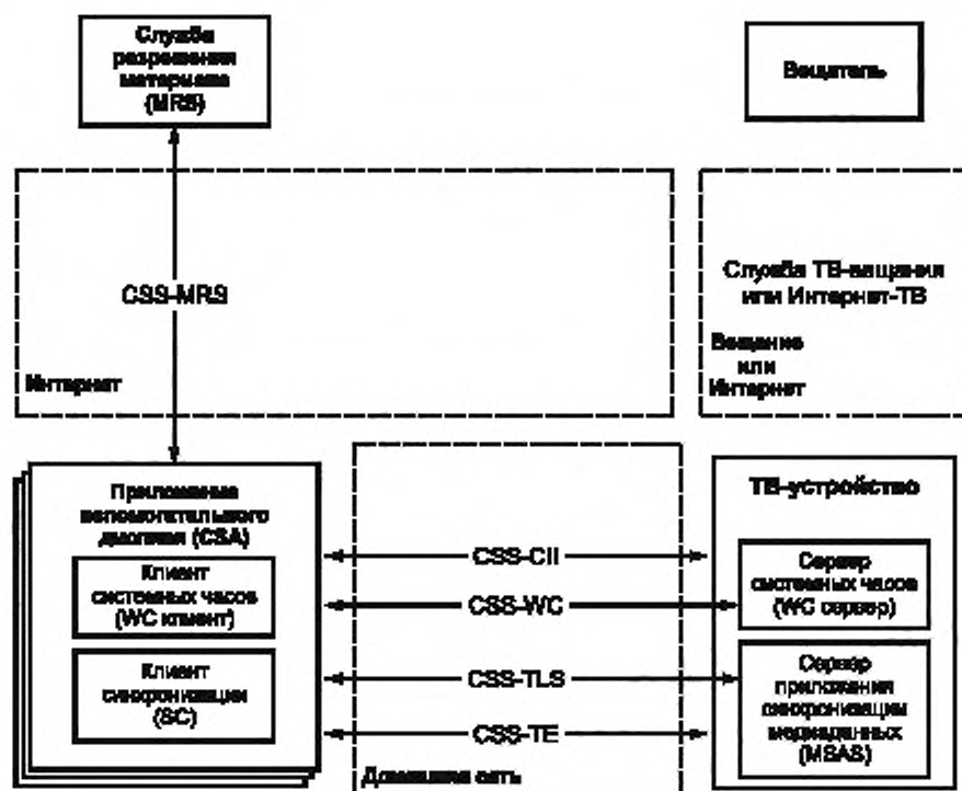
Рисунок 4 — Интерфейсы идентификации контента и синхронизации медиаданных
