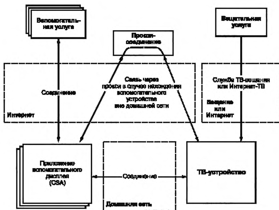
Рисунок 2 — Базовая архитектура составной предоставляемой услуги
