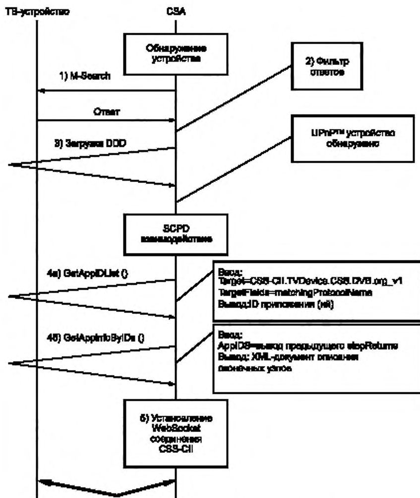
Рисунок 6 — Последовательность команд между CSSA и ТВ-устройством для установления WebSocket соединения CII
