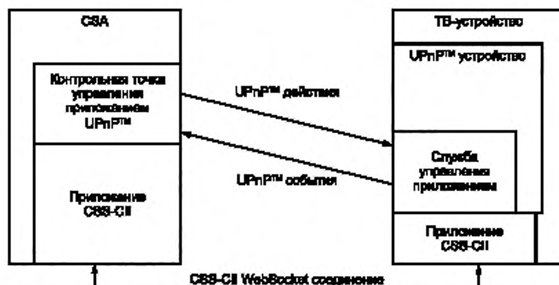
Рисунок 5 — CSA и ТВ-устройство, реализующее управление приложением UPnP™ и связи приложения CII
