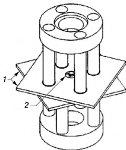
1 — пластина; 2 — болт
