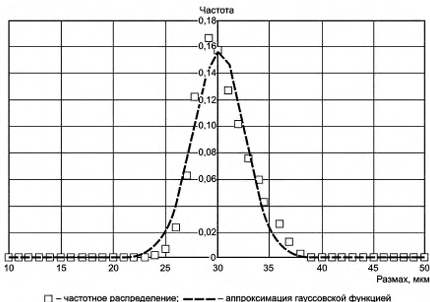
Рисунок 6 — Частотное распределение размаха и его аппроксимация гауссовской функцией
