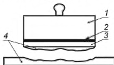
в) AT-3 — отрыв по телу основания
