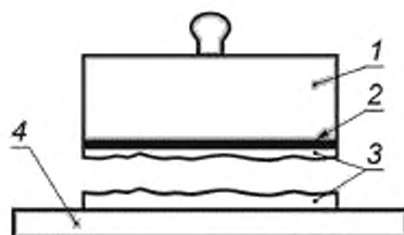
б) AT-2 — разрыв по телу образца (когезионный отрыв)
