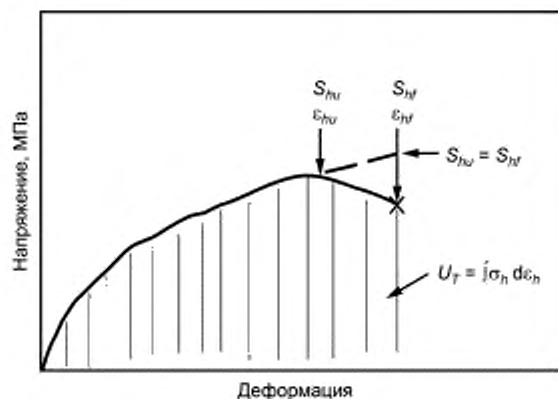
S_{hu} — предел прочности при растяжении в окружном направлении; S_{hf} — предел прочности при разрыве в окружном направлении; U_T — удельная работа растяжения
