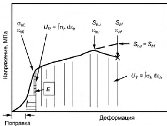
\sigma_{n0} — напряжение на пределе пропорциональности; \epsilon_{n0} — деформация на пределе пропорциональности; S_{hu} — предел прочности при растяжении в окружном направлении; S_{hf} — предел прочности при разрыве в окружном направлении; U_R — удельная потенциальная энергия растяжения, U_T — удельная работа растяжения; E — модуль упругости при растяжении
