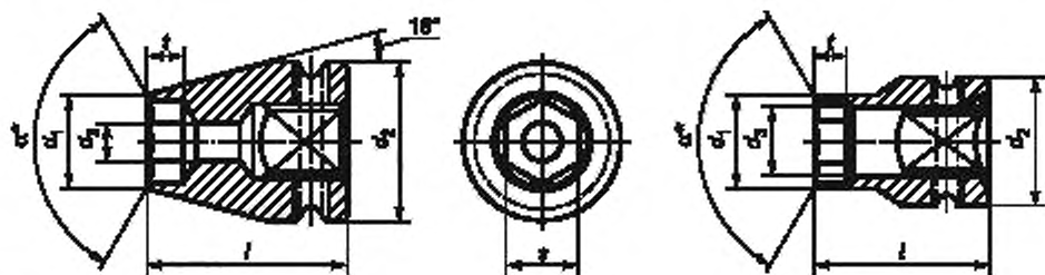
Рисунок 4 — Сменные головки с d_1 < d_2
