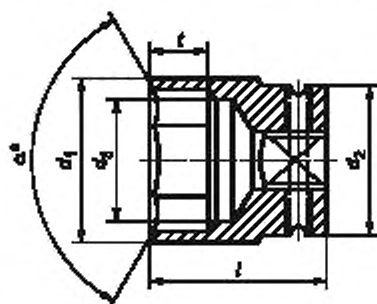
Рисунок 6 — Сменные головки с d_1 > d_2
