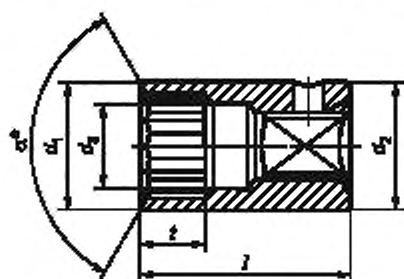
Рисунок 1 — Сменные головки с d_1 < d_2
