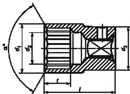
Рисунок 3 — Сменные головки с d_1 > d_2
