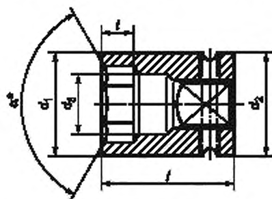
Рисунок 5 — Сменные головки с d_1 = d_2
