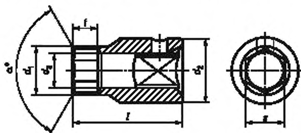
Рисунок 1 — Сменные головки с d_1 < d_2
