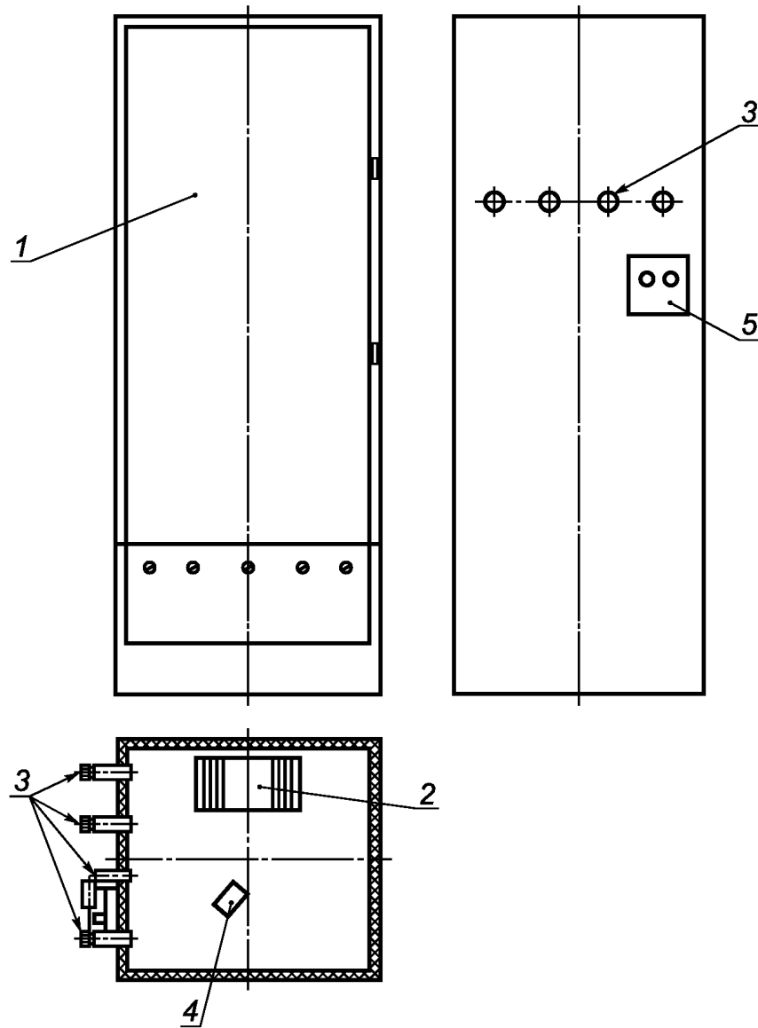
1 — термощкаф; 2 — нагревательный элемент; 3 — штуцера отбора проб; 4 — термодатчик; 5 — блок управления
