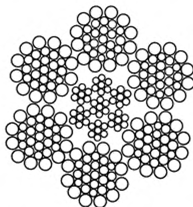
Шестипрядный канат 6×31+1 м. с.; 6×31=186 проволок с металлическим сердечником конструкции 7×7=49 проволок (прядь каната 1+6+6/6+12; прядь сердечника 1+6).
