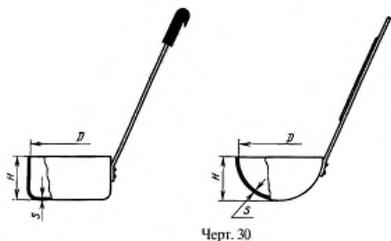
Ложка разливательная
