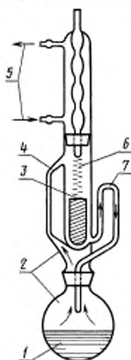
1 — растворитель; 2 — восходящий пар; 3 — экстракционная гильза с веществом; 4 — паровая труба; 5 — охлаждающая вода; 6 — конденсированный растворитель; 7 — раствор
