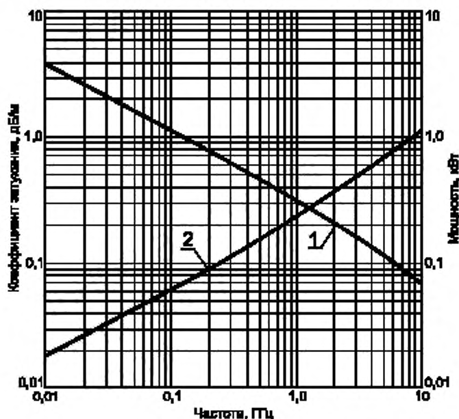
Частотные зависимости
