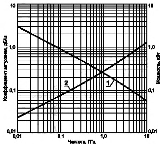
Частотные зависимости
