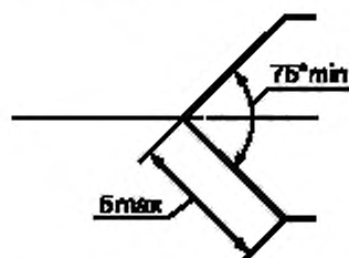
Рисунок 1 — Угол схождения боковых граней острья клинка
