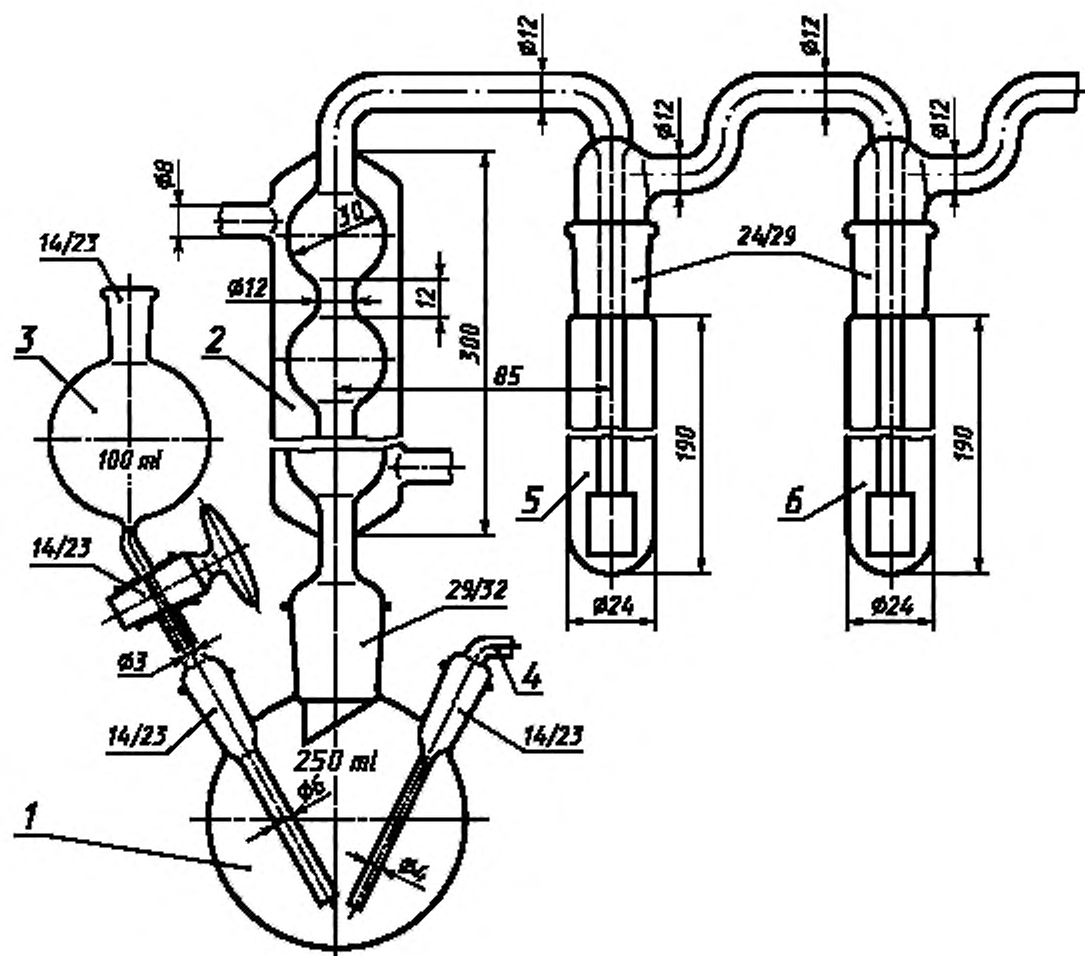
1 — дистилляционная колба; 2 — обратный холодильник; 3 — капельная воронка; 4 — подводящая трубка; 5 и 6 — газопоглотительные устройства
