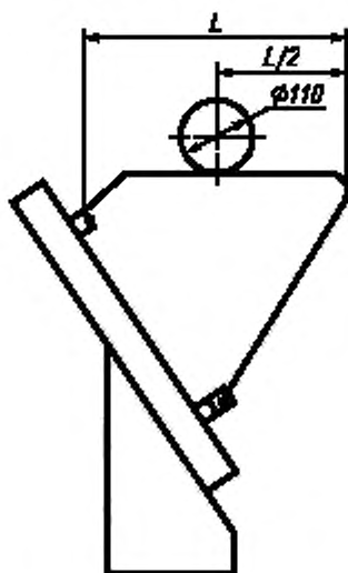
Рисунок 1 — Испытания на вертикальную нагрузку
