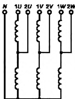
Рисунок Ж.7 — Маркировка трехфазного автотрансформатора ( Y_n \text{ авто}/D-0 )
