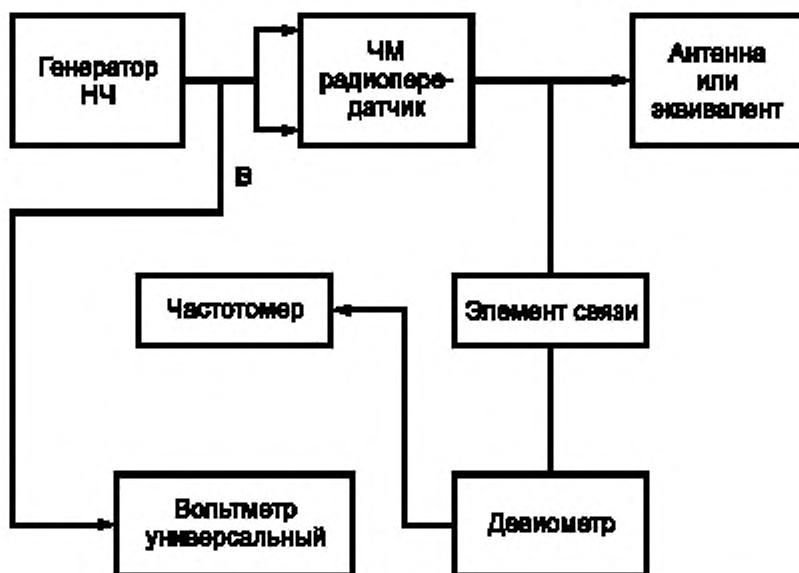
Рисунок 1 — Схема измерений параметров систем стереофонического радиовещания
