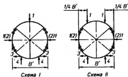
г) Кольцевые кресты
