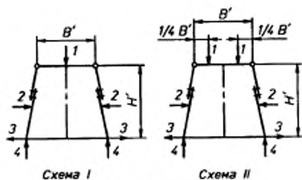
а) Трапециевидные кресты
