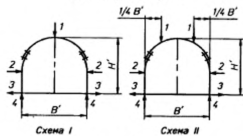
а) Трёхзвенные арочные крепи
